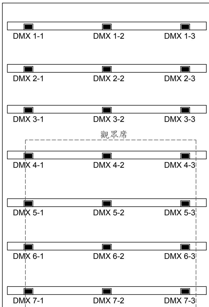
DMX 訊號孔位置圖
